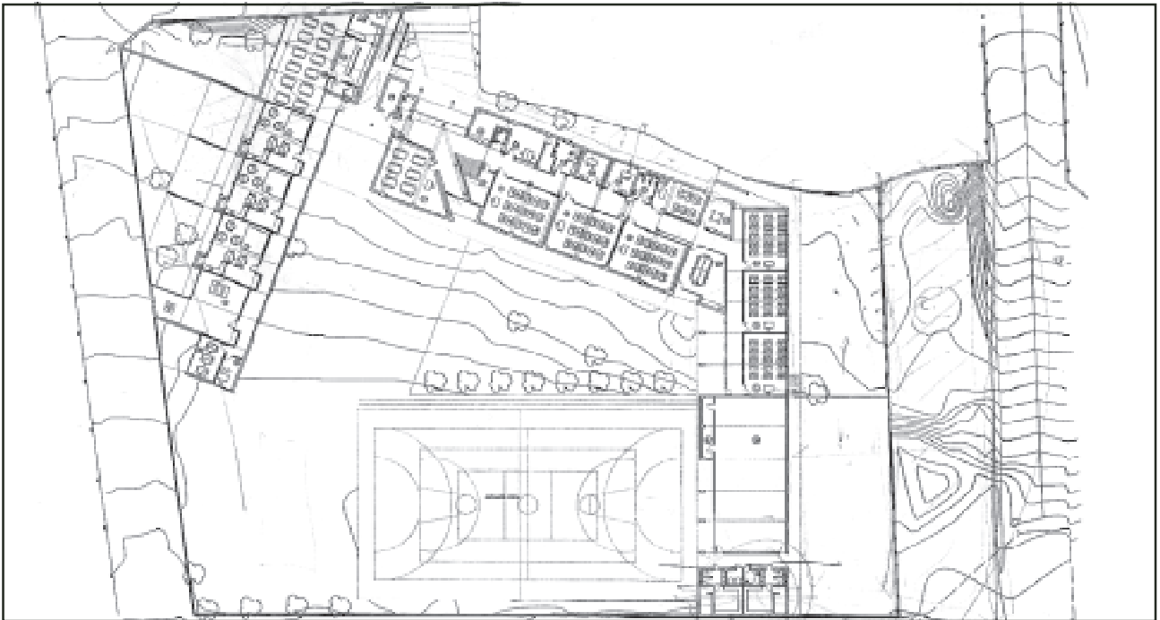
Plànol d'ampliació de l'escola, planta baixa
