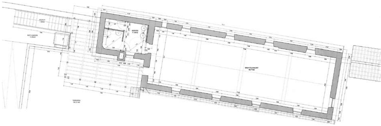
PLÀNOL DE LA PRIMERA PLANTA DE LA REHABILITACIÓ DEL CORRAL DE LA FARGA
